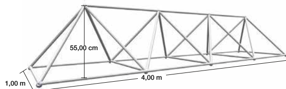
Χωροδικτύωμα
