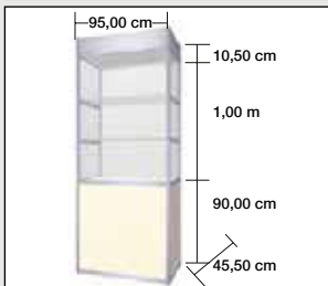
Βιτρίνα όψεως
